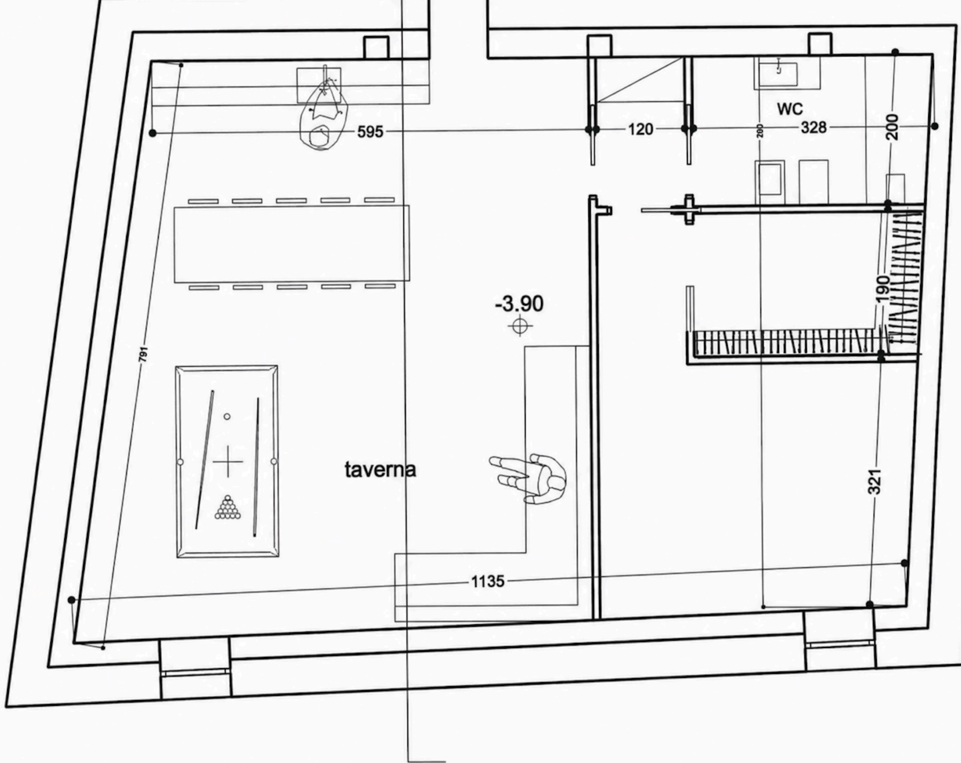
PIANTA PIANO INTERRATO STATO IN PROGETTO
