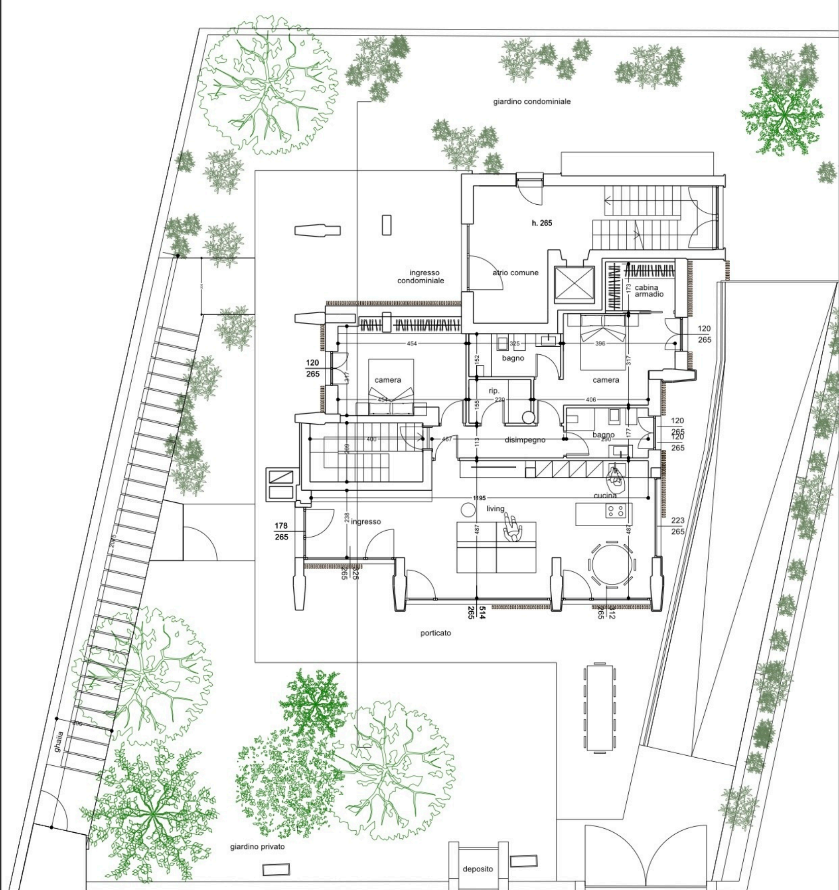
PIANTA PIANO TERRA STATO IN PROGETTO
